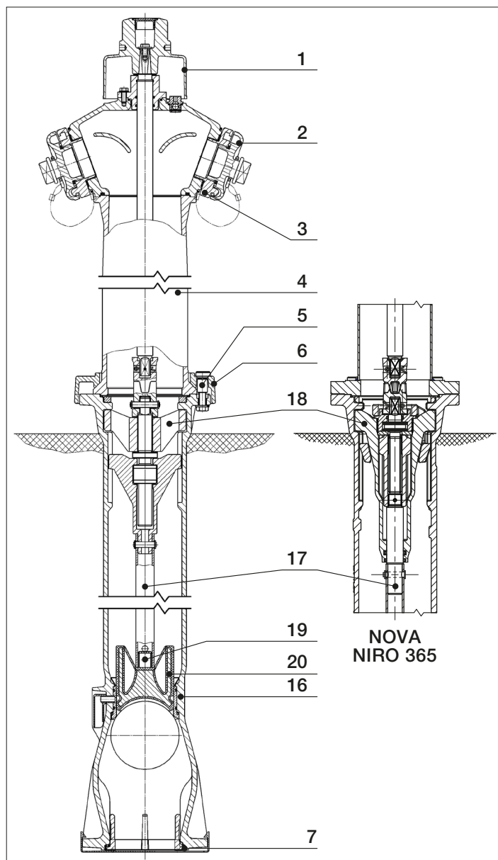
Obr. 5.: Schéma hydrantu
